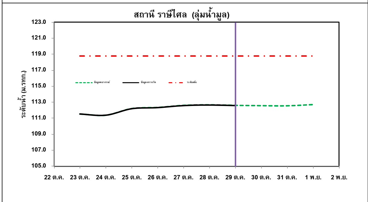
รูปที่ ๕ กราฟการพยากรณ์ระดับน้ำจุดสำคัญในพื้นที่ลุ่มน้ำมูล
