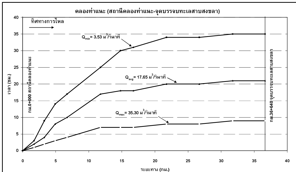
รูปที่ 5 ระยะเวลาการเดินทางของน้ำที่ค่าอัตราการไหลในปริมาณสูง ปานกลาง และต่ำ ของคลองทำแนะ
