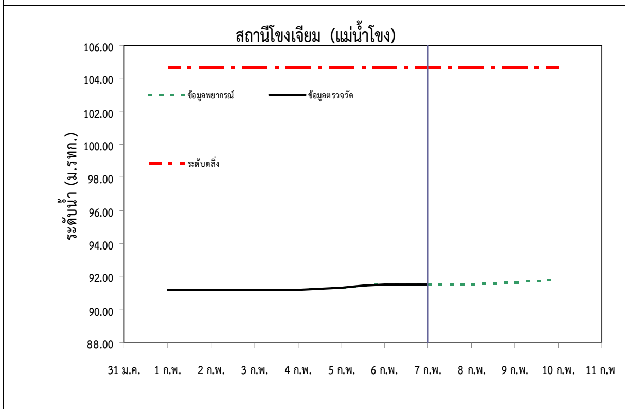
รูปที่ 2 กราฟการพยากรณ์ระดับน้ำจุดสำคัญในแม่น้ำโขง (ต่อ)
