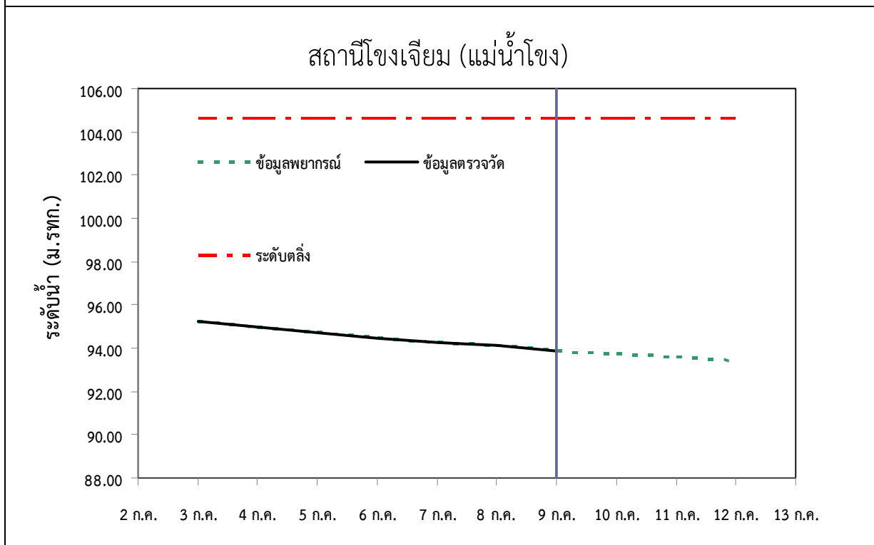
รูปที่ 2 กราฟการพยากรณ์ระดับน้ำจุดสำคัญในแม่น้ำโขง (ต่อ)
