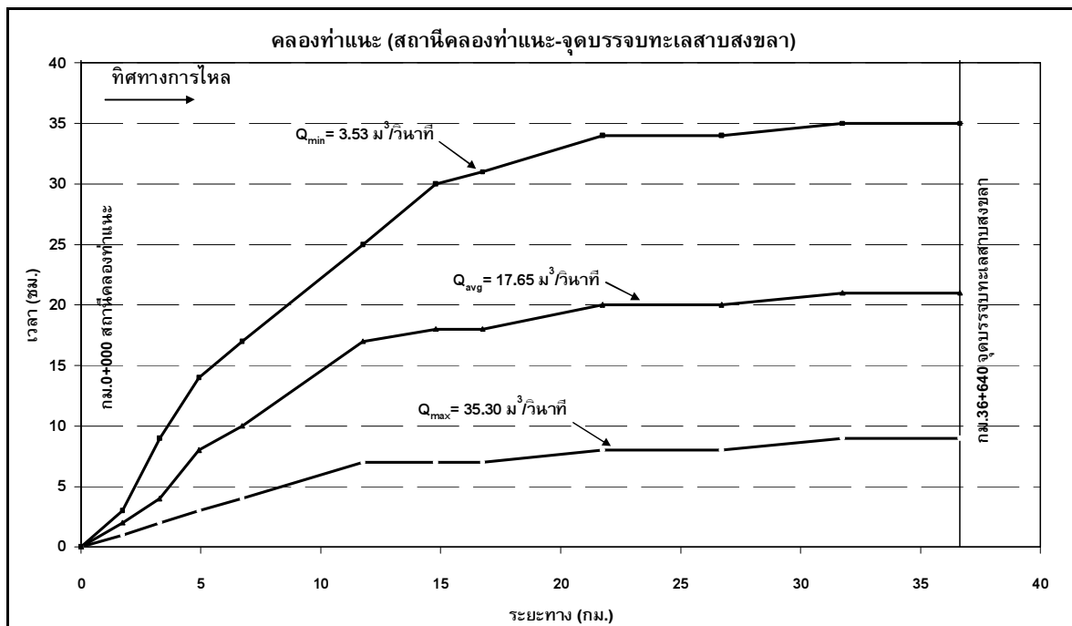
รูปที่ 5 ระยะเวลาการเดินทางของน้ำที่ค่าอัตราการไหลในปริมาณสูง ปานกลาง และต่ำ ของคลองทำนวะ
