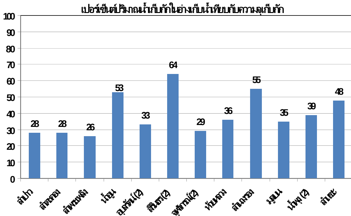
รูปที่ ๑๒ กราฟแสดงเปอร์เซ็นต์ปริมาณน้ำในอ่างเทียบกับความจุเก็บกักของอ่างขนาดใหญ่
