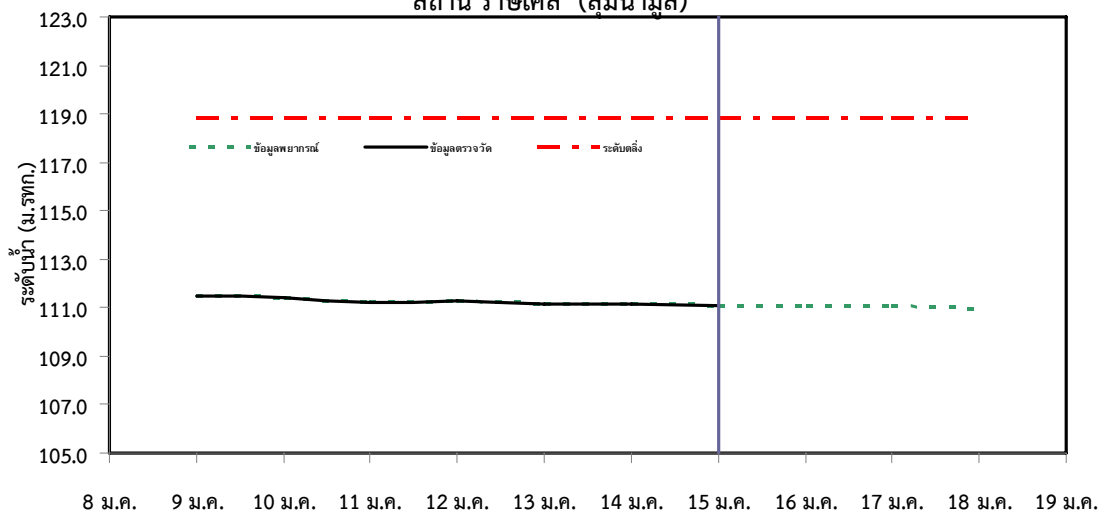
รูปที่ 5 กราฟการพยากรณ์ระดับน้ำจุดสำคัญในพื้นที่ลุ่มน้ำมูล
