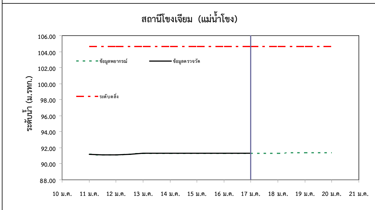
รูปที่ 2 กราฟการพยากรณ์ระดับน้ำจุดสำคัญในแม่น้ำโขง (ต่อ)
