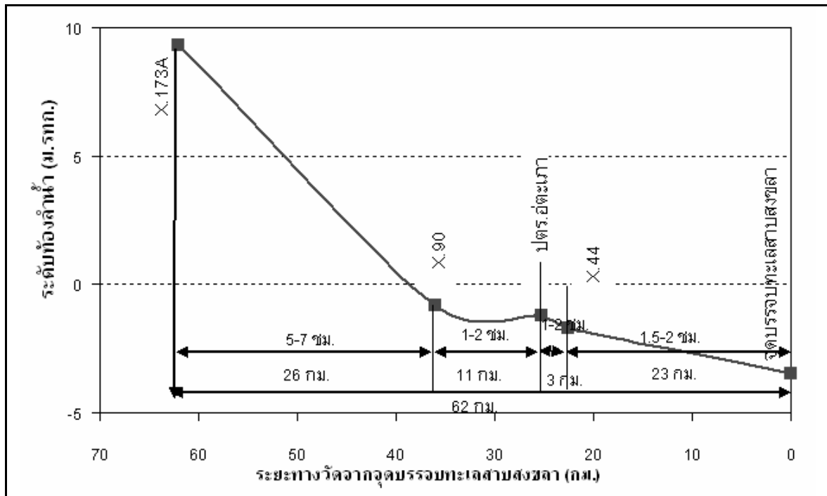
รูปที่ 4 รูปตัดตามยาวและเวลาการเดินทางของน้ำในคลองอุตะเถาตั้งแต่ สถานีน้ำท่า X.173A ถึงจุดบรรจบทะเลสาบสงขลา
