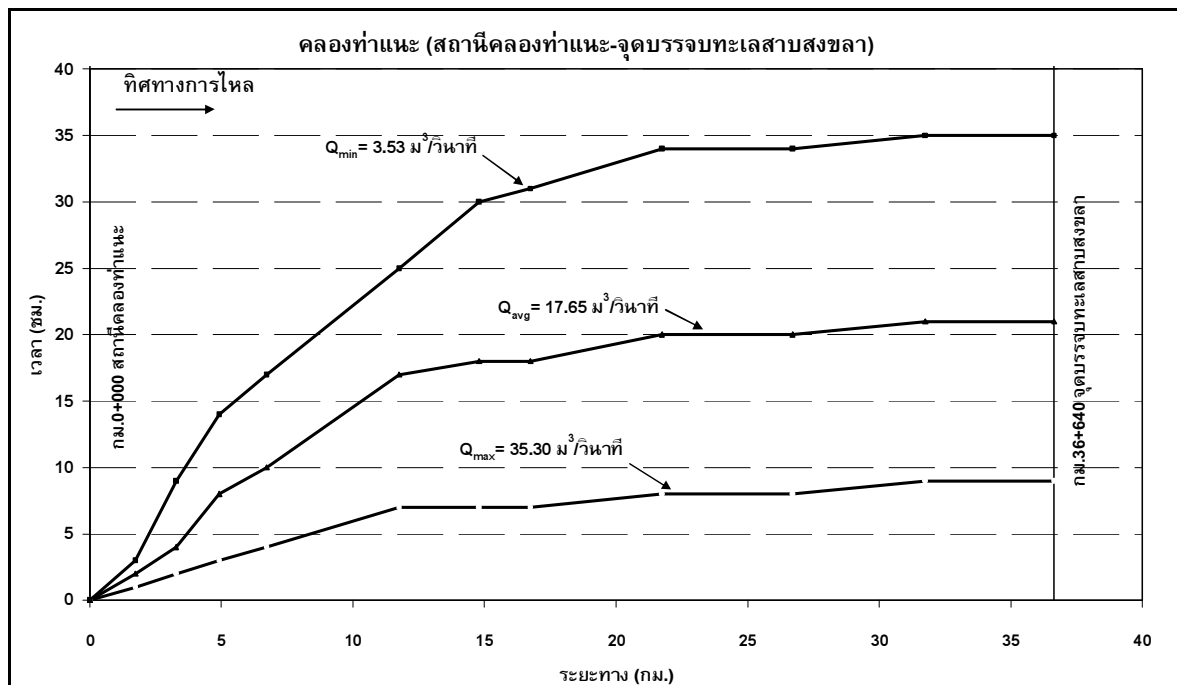
รูปที่ 5 ระยะเวลาการเดินทางของน้ำที่ค่าอัตราการไหลในปริมาณสูง ปานกลาง และต่ำ ของคลองทำนง
