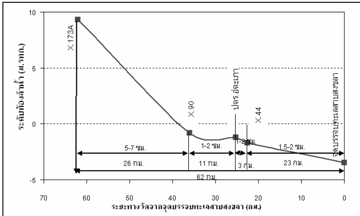
รูปที่ 4 รูปตัดตามยาวและเวลาการเดินทางของน้ำในคลองอยู่ตะเภาดั้งแต่ สถานีน้ำที่ X.173A ถึงจุดบรรจบทะเลสาบสงขลา
