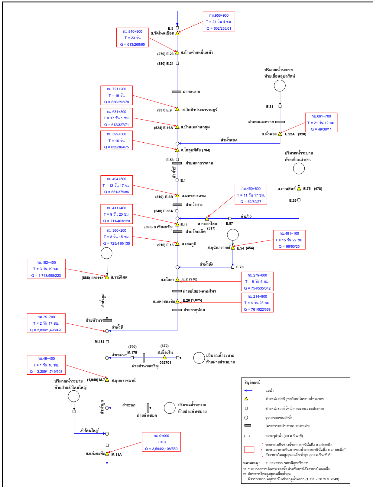
รูปที่ 11 แสดงแผนภูมิของโครงข่ายแม่น้ำความจุลำนํ้า และระยะเวลาเดินทางของน้ำ
