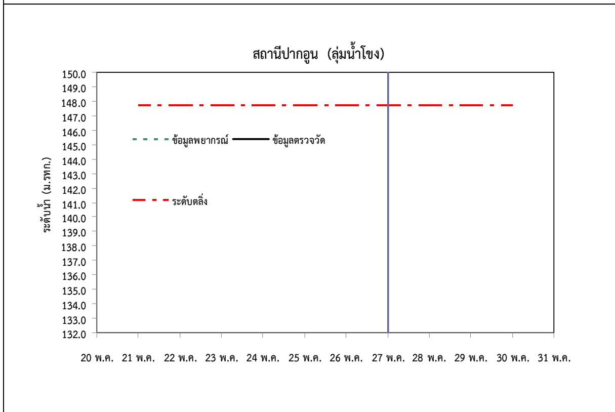
รูปที่ 3 กราฟการพยากรณ์ระดับน้ำจุดสำคัญในพื้นที่ลุ่มน้ำโขง (ต่อ)
