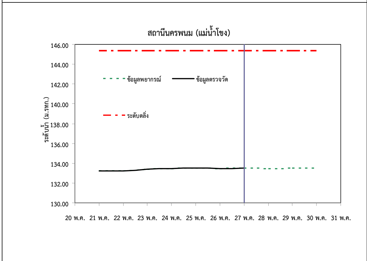
รูปที่ 2 กราฟการพยากรณ์ระดับน้ำจุดสำคัญในแม่น้ำโขง
