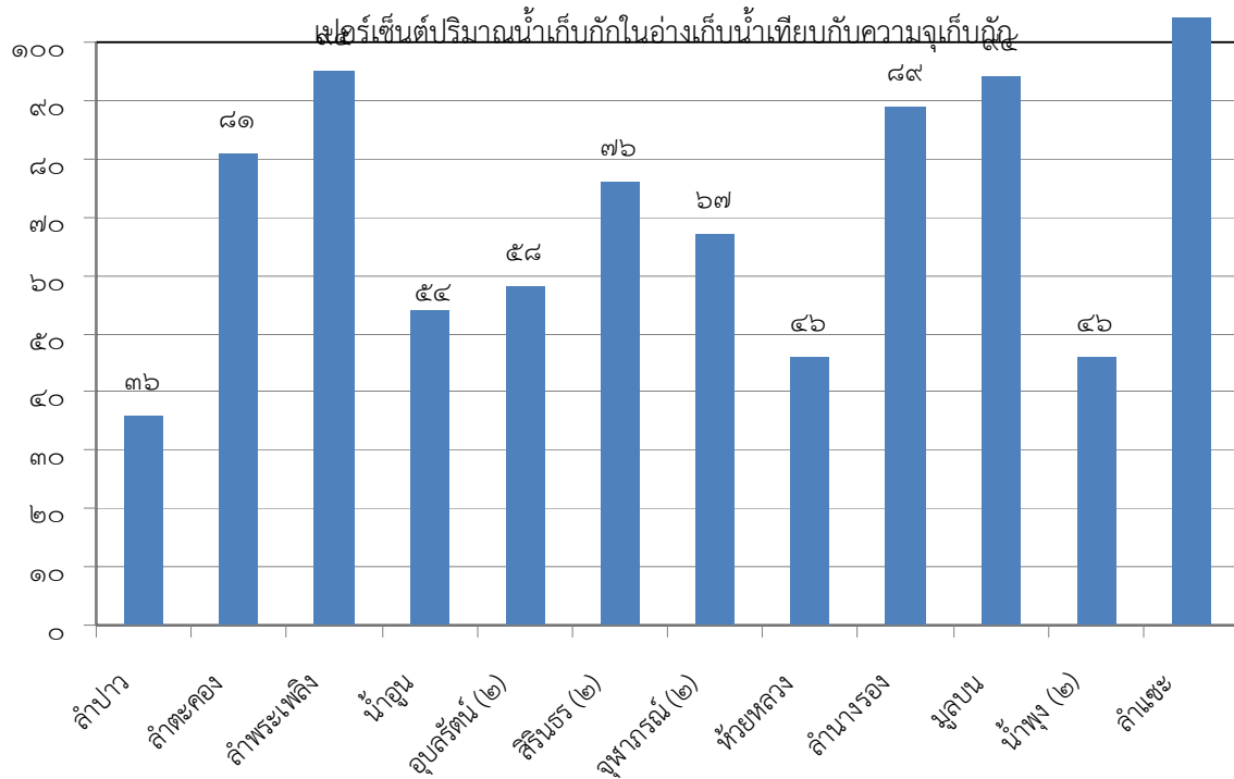
รูปที่ ๑๒ กราฟแสดงเปอร์เซ็นต์ปริมาณน้ำในอ่างเทียบกับความจุเก็บกักของอ่างขนาดใหญ่
