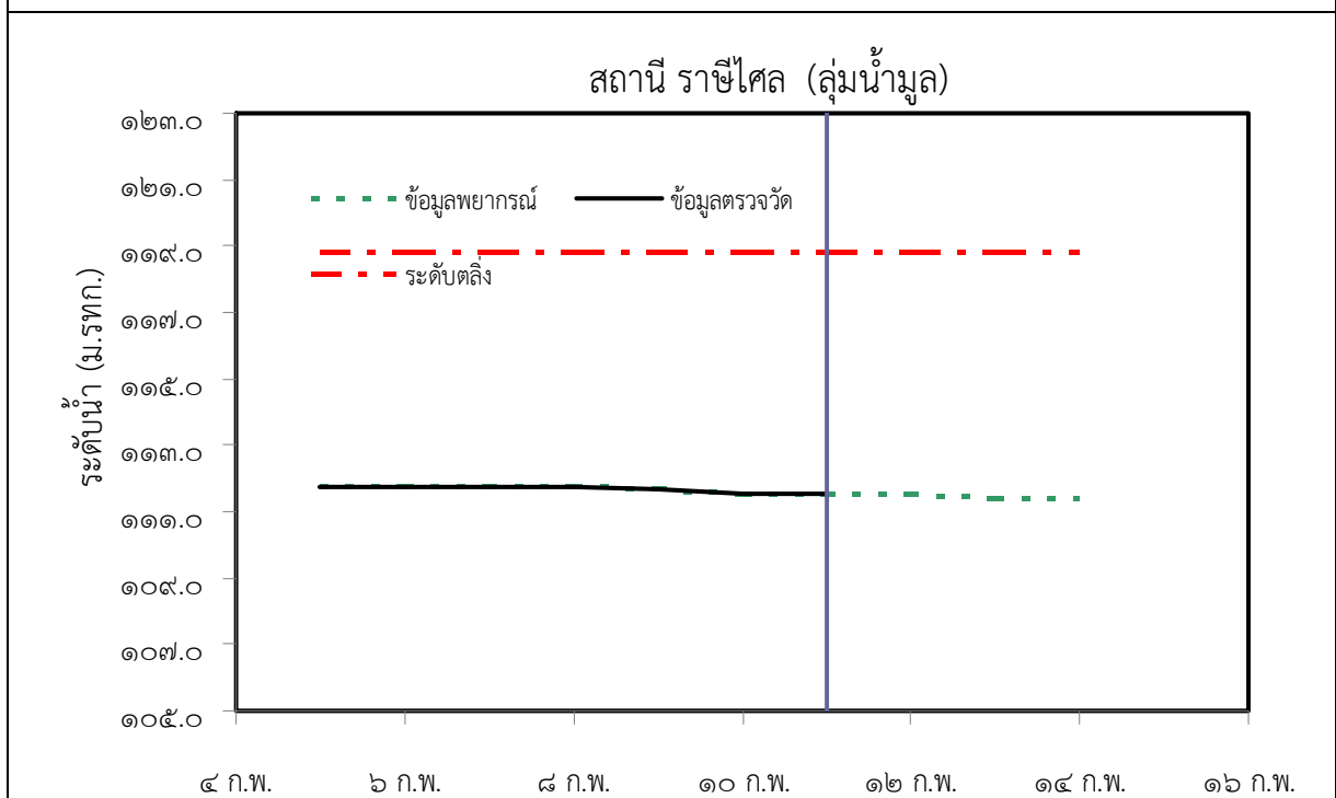
รูปที่ ๕ กราฟการพยากรณ์ระดับน้ำจุดสำคัญในพื้นที่ลุ่มน้ำมูล
