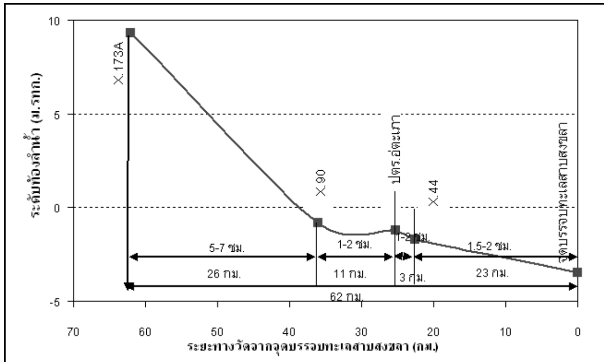
รูปที่ 4 รูปตัดตามยาวและเวลาการเดินทางของน้ำในคลองอุต๊ะเกาตั้งแต่ สถานีน้ำท่า X.173A ถึงจุดบรรจบทะเลสาบสงขลา
