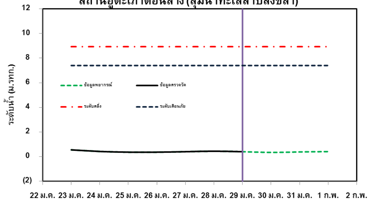
รูปที่ 2 กราฟการพยากรณ์ระดับน้ำจุดสำคัญในพื้นที่ลุ่มน้ำทะเลสาบสงขลา
