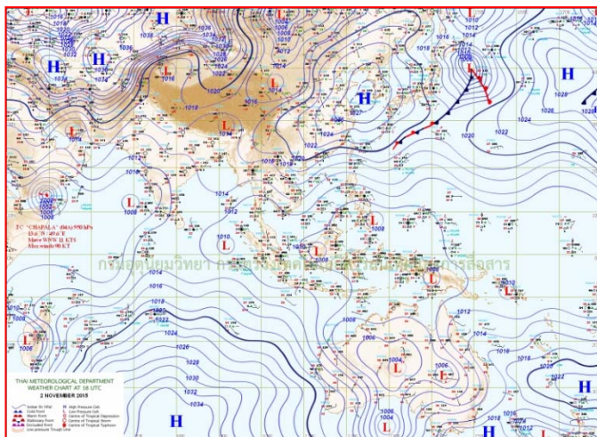
แผนที่อากาศ วันที่ ๓ พ.ย. ๒๕๕๘ เวลา ๐๖.๐๐ น.
