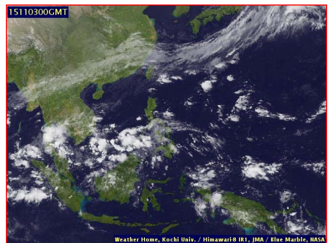
ภาพถ่ายจากดาวเทียม วันที่ ๓ พ.ย. ๒๕๕๘ เวลา ๐.๐๐ น.
