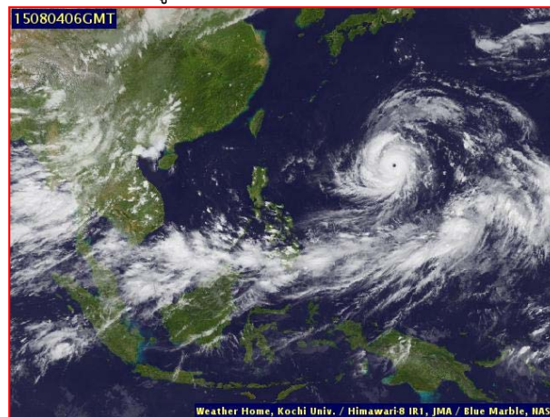
ภาพถ่ายจากดาวเทียม วันที่ ๔ ส.ค. ๒๕๕๘ เวลา ๑๓.๐๐ น.
