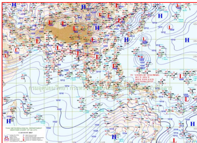
แผนที่อากาศ วันที่ ๔ ส.ค. ๒๕๕๘ เวลา ๐๗.๐๐ น.
