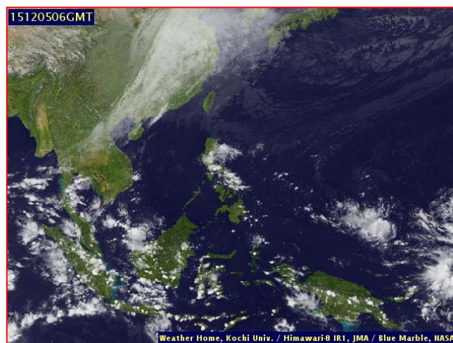
ภาพถ่ายจากดาวเทียม วันที่ ๕ ธ.ค. ๒๕๕๘ เวลา ๑๓.๐๐ น.
