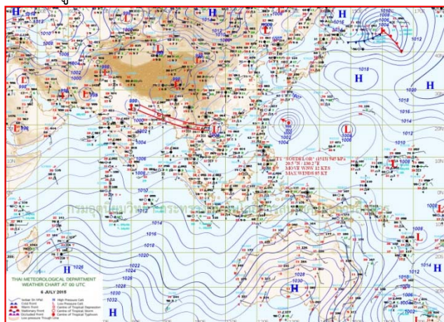
แผนที่อากาศ วันที่ ๖ ส.ค. ๒๕๕๘ เวลา ๐๗.๐๐ น.
