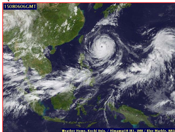
ภาพถ่ายจากดาวเทียม วันที่ ๖ ส.ค. ๒๕๕๘ เวลา ๑๓.๐๐ น.
