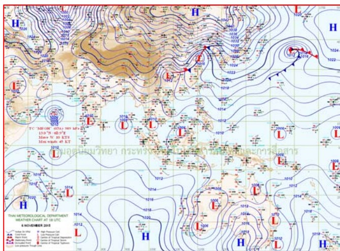
แผนที่อากาศ วันที่ ๗ พ.ย. ๒๕๕๘ เวลา ๐๖.๐๐ น.
