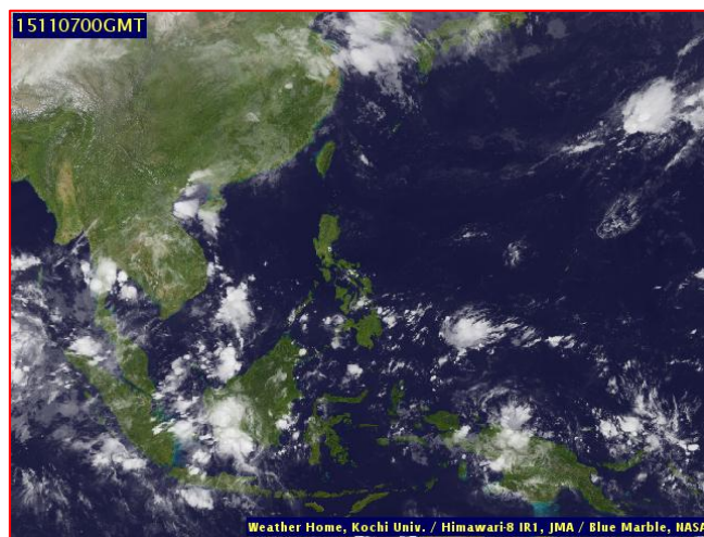
ภาพถ่ายจากดาวเทียม วันที่ ๗ พ.ย. ๒๕๕๘ เวลา ๐๗.๐๐ น.
