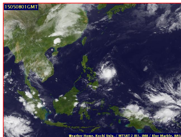
ภาพถ่ายจากดาวเทียม วันที่ 8 พ.ค. 2558
