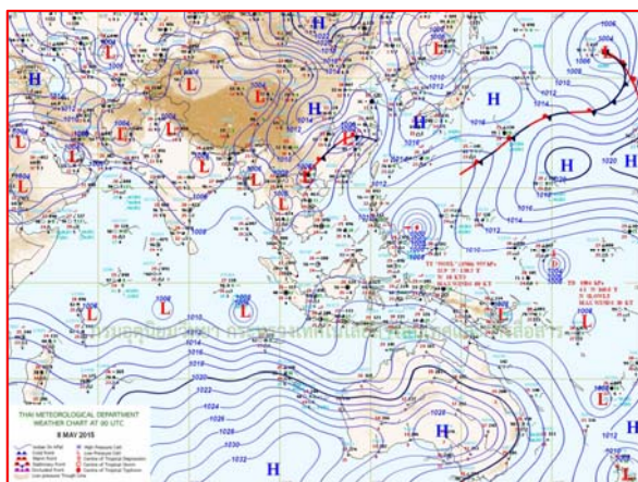
แผนที่อากาศ วันที่ 8 พ.ค. 2558 เวลา 07.00 น.
