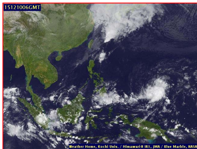
ภาพถ่ายจากดาวเทียม วันที่ ๑๐ ธ.ค. ๒๕๕๘ เวลา ๑๓.๐๐ น.
