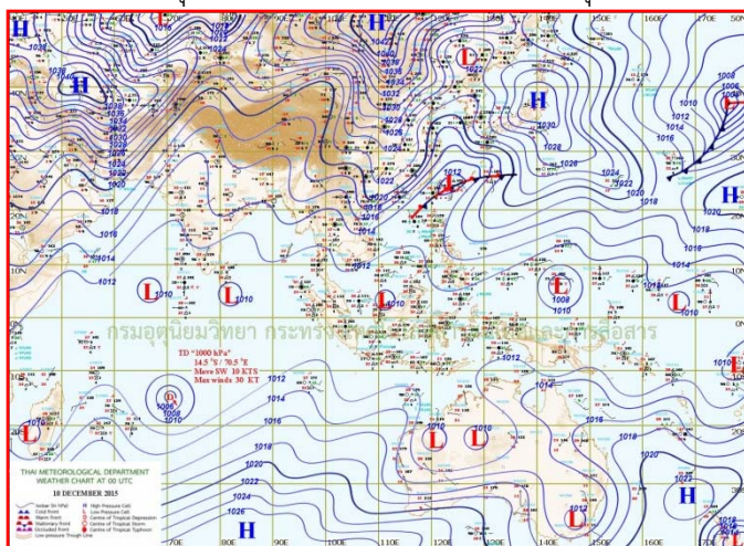
แผนที่อากาศ วันที่ ๑๐ ธ.ค. ๒๕๕๘ เวลา ๐๗.๐๐ น.
