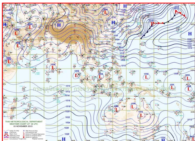
แผนที่อากาศ วันที่ ๑๑ พ.ย. ๒๕๕๘ เวลา ๐๑.๐๐ น.
