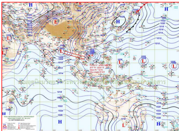
แผนที่อากาศ วันที่ ๑๔ ก.ย. ๒๕๕๘ เวลา ๐๑.๐๐ น.
