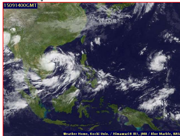
ภาพถ่ายจากดาวเทียม วันที่ ๑๔ ก.ย. ๒๕๕๘ เวลา ๐๗.๐๐ น.
