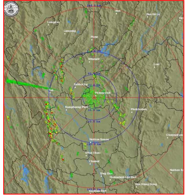
สถานีสุราษฎร์ธานี เวลา ๐๘.๓๐ น.
