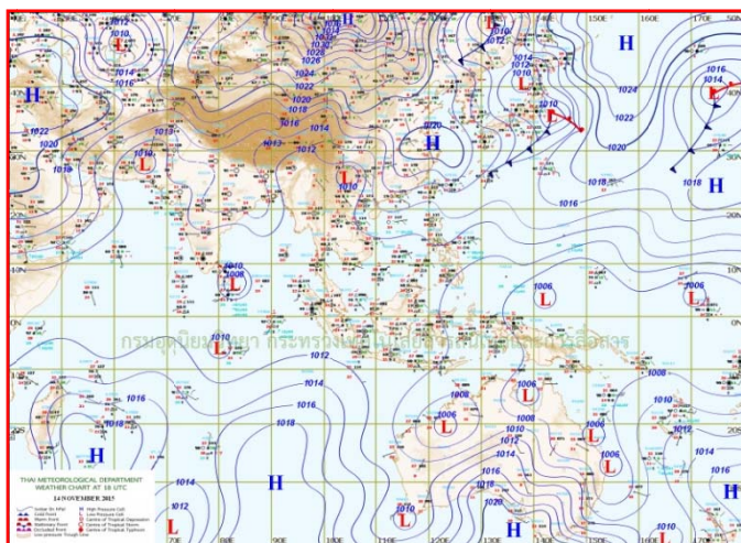
แผนที่อากาศ วันที่ ๑๕ พ.ย. ๒๕๕๘ เวลา ๐๖.๐๐ น.
