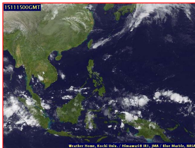
ภาพถ่ายจากดาวเทียม วันที่ ๑๕ พ.ย. ๒๕๕๘ เวลา ๐๗.๐๐ น.
