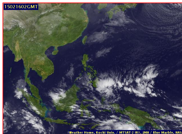
ภาพถ่ายจากดาวเทียม วันที่ 16 ก.พ. 2558
