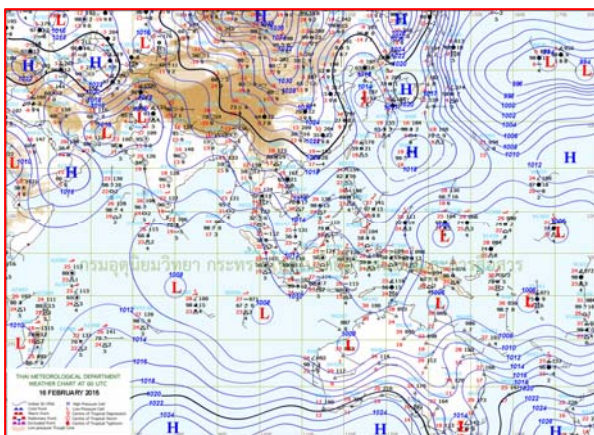
แผนที่อากาศ วันที่ 16 ก.พ. 2558 เวลา 07.00 น.
