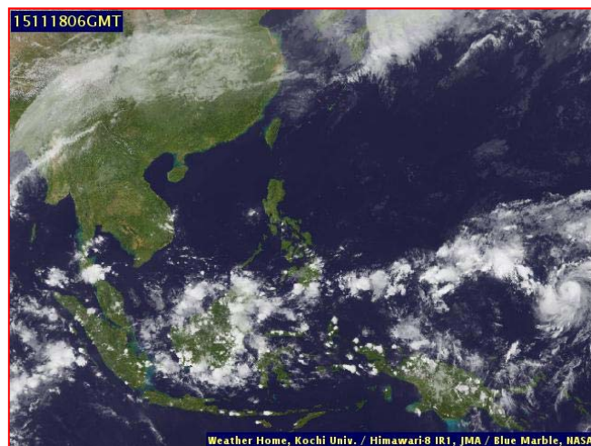
ภาพถ่ายจากดาวเทียม วันที่ ๑๘ พ.ย. ๒๕๕๘ เวลา ๑๓.๐๐ น.
