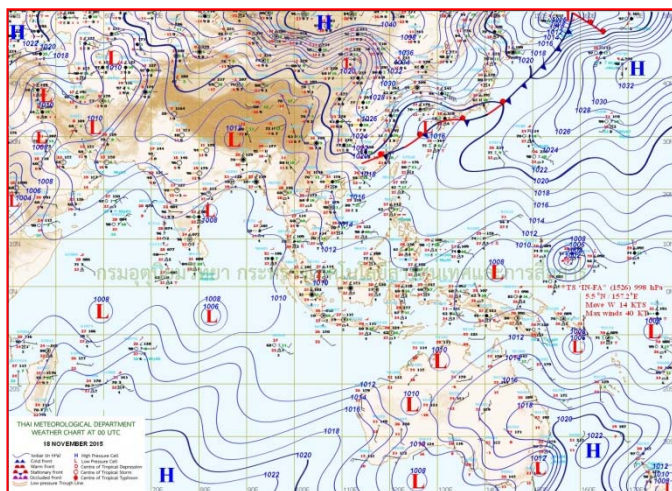
แผนที่อากาศ วันที่ ๑๘ พ.ย. ๒๕๕๘ เวลา ๐๗.๐๐ น.
