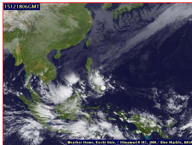
ภาพถ่ายจากดาวเทียม วันที่ ๑๘ ธ.ค. ๒๕๕๘ เวลา ๑๓.๐๐ น.
