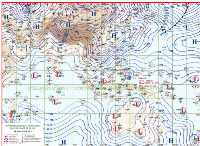
แผนที่อากาศ วันที่ ๑๘ ธ.ค. ๒๕๕๘ เวลา ๐๗.๐๐ น.
