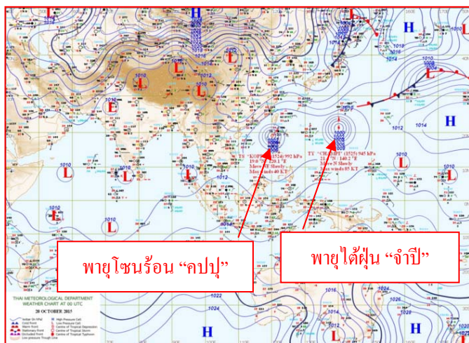
แผนที่อากาศ วันที่ ๒๐ ต.ค. ๒๕๕๘ เวลา ๐๗.๐๐ น.
