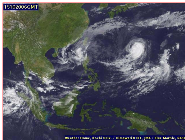
ภาพถ่ายจากดาวเทียม วันที่ ๒๐ ต.ค. ๒๕๕๘ เวลา ๑๓.๐๐ น.
