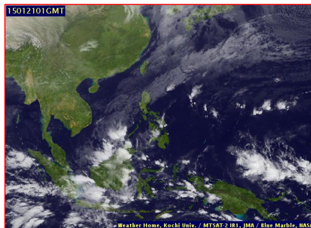
ภาพถ่ายจากดาวเทียม วันที่ 21 ม.ค. 2558
