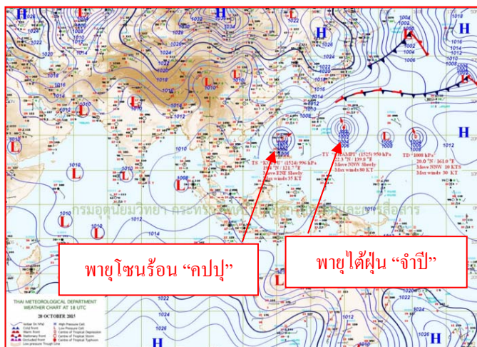
แผนที่อากาศ วันที่ ๒๑ ต.ค. ๒๕๕๘ เวลา ๐๑.๐๐ น.
