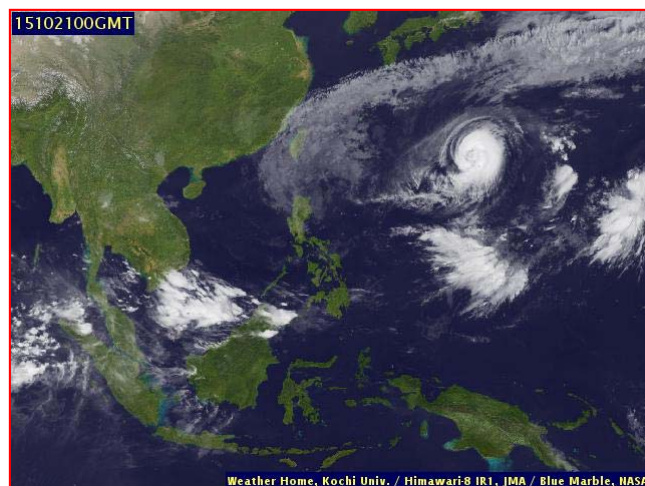
ภาพถ่ายจากดาวเทียม วันที่ ๒๑ ต.ค. ๒๕๕๘ เวลา ๐๘.๐๐ น.
