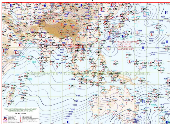
แผนที่อากาศ วันที่ ๒๖ ก.ค. ๒๕๕๘ เวลา ๐๑.๐๐ น.
