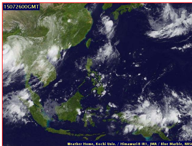
ภาพถ่ายจากดาวเทียม วันที่ ๒๖ ก.ค. ๒๕๕๘ เวลา ๐๗.๐๐ น.
