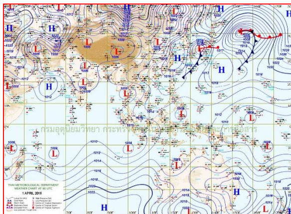
แผนที่อากาศ วันที่ 1 เม.ย. 2559 เวลา 07.00 น.
