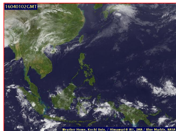
ภาพถ่ายจากดาวเทียม วันที่ 1 เม.ย. 2559
