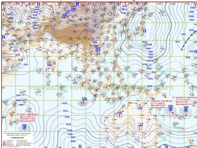
แผนที่อากาศ วันที่ ๑๒ ก.พ. ๒๕๕๙ เวลา ๐๗.๐๐ น.
