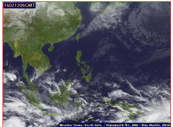
ภาพถ่ายจากดาวเทียม วันที่ ๑๒ ก.พ. ๒๕๕๙ เวลา ๑๓.๐๐ น.
