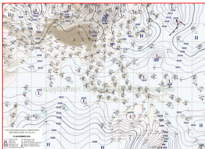
แผนที่อากาศ วันที่ ๑๓ พ.ย. ๒๕๕๙ เวลา ๐๗.๐๐ น.
