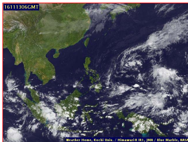
ภาพถ่ายจากดาวเทียม วันที่ ๑๓ พ.ย. ๒๕๕๙ เวลา ๑๓.๐๐ น.
