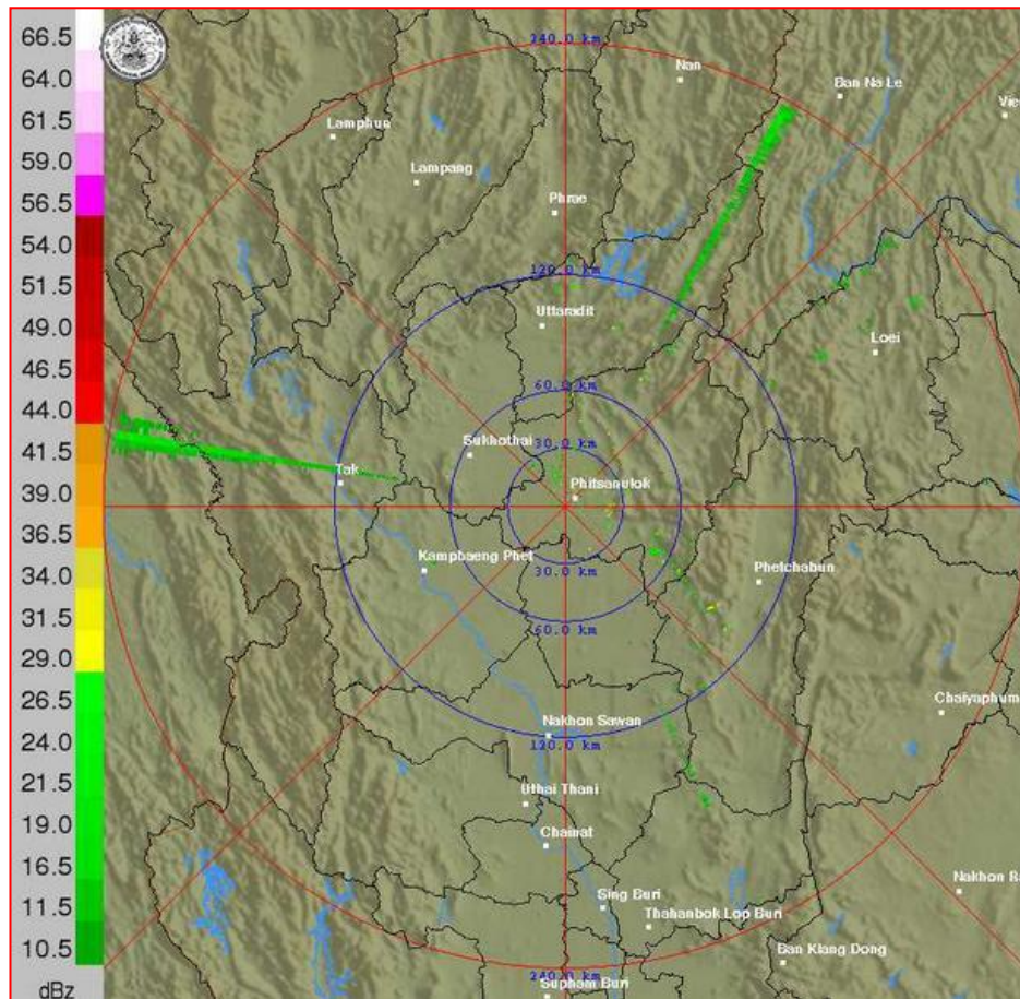
ภาพเรดาร์ตรวจอากาศ “พิษณุโลก” ณ วันที่ 15 ธันวาคม 2559 (ที่มา : กรมอุตุนิยมวิทยา)
