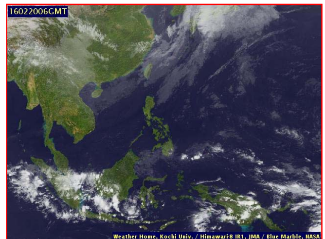
ภาพถ่ายจากดาวเทียม วันที่ ๒๐ ก.พ. ๒๕๕๙ เวลา ๑๓.๐๐ น.
