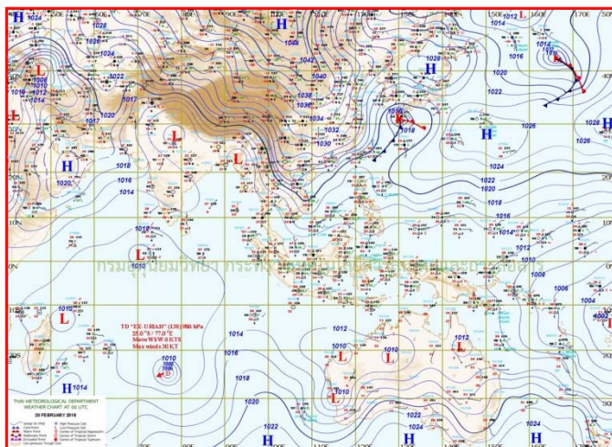
แผนที่อากาศ วันที่ ๒๐ ก.พ. ๒๕๕๙ เวลา ๐๗.๐๐ น.
