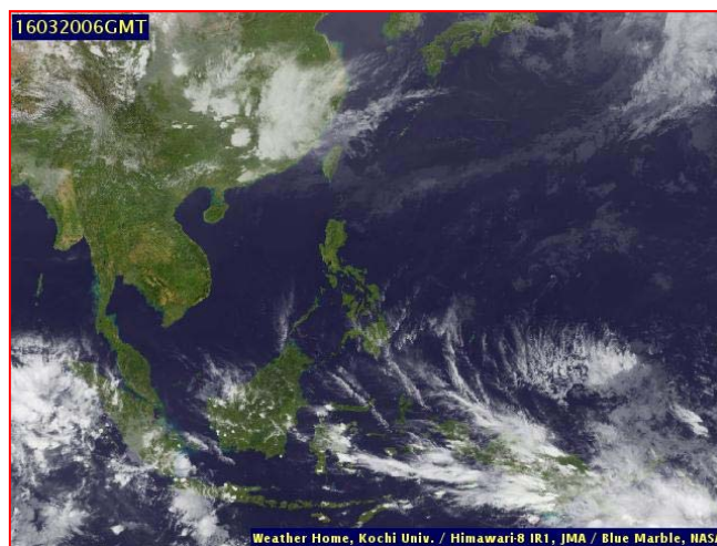
ภาพถ่ายจากดาวเทียม วันที่ ๒๐ มี.ค. ๒๕๕๙ เวลา ๑๓.๐๐ น.
