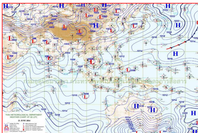
แผนที่อากาศ วันที่ ๒๑ มิ.ย.๒๕๕๙ เวลา ๐๗.๐๐ น.
