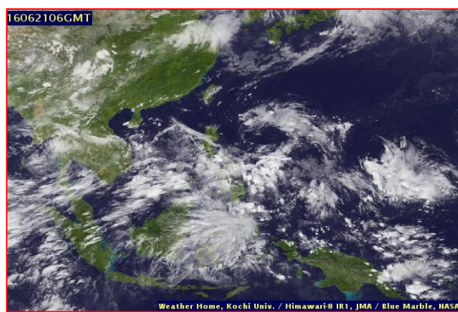
ภาพถ่ายจากดาวเทียม วันที่ ๒๑ มิ.ย. ๒๕๕๙ เวลา ๑๓.๐๐ น.
