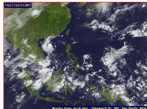
ภาพถ่ายจากดาวเทียม วันที่ 26 ก.ค. 2559
