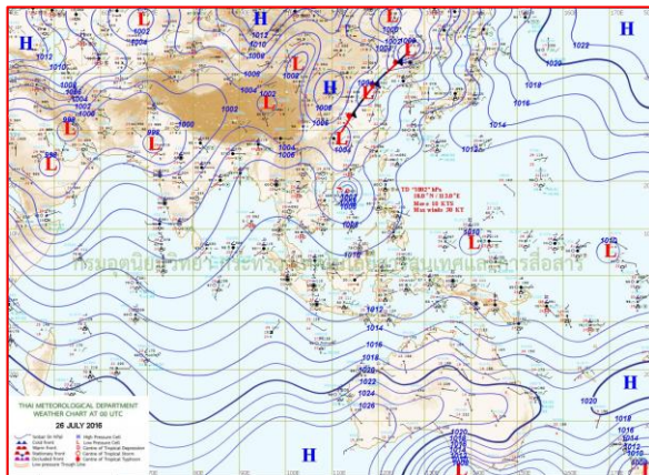
แผนที่อากาศ วันที่ 26 ก.ค. 2559 เวลา 07.00 น.
