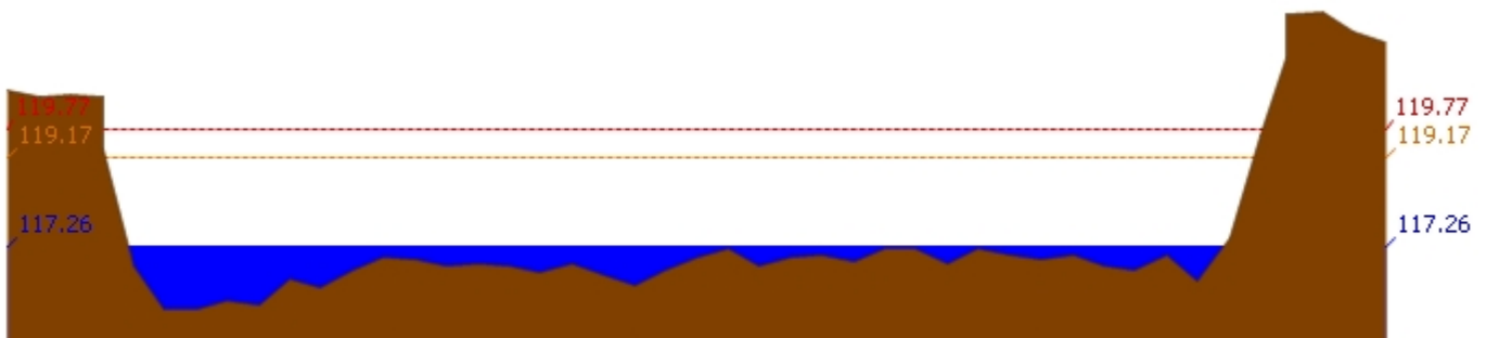
สถานี 060111T แม่น้ำปิงที่บ้านปากร่องห้วยจี้ ต.ตากออก อ.บ้านตาก จ.ตาก ระดับน้ำ 117.26 ม.รทก.
