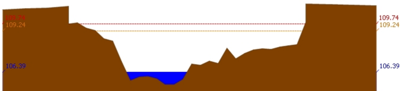
สถานี 061701T ห้วยแม่ท้อที่อำเภอเมืองตาก ค.แม่ท้อ อ.เมืองตาก จ.ตาก ระดับน้ำ 106.39 ม.รทก.
