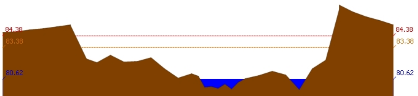
สถานี 062001T คลองสวนหมากที่บ้านน้ำไทรง ต.ท่าขุนราม อ.เมือง จ.กำแพงเพชร ระดับน้ำ 80.62 ม.รทก.
