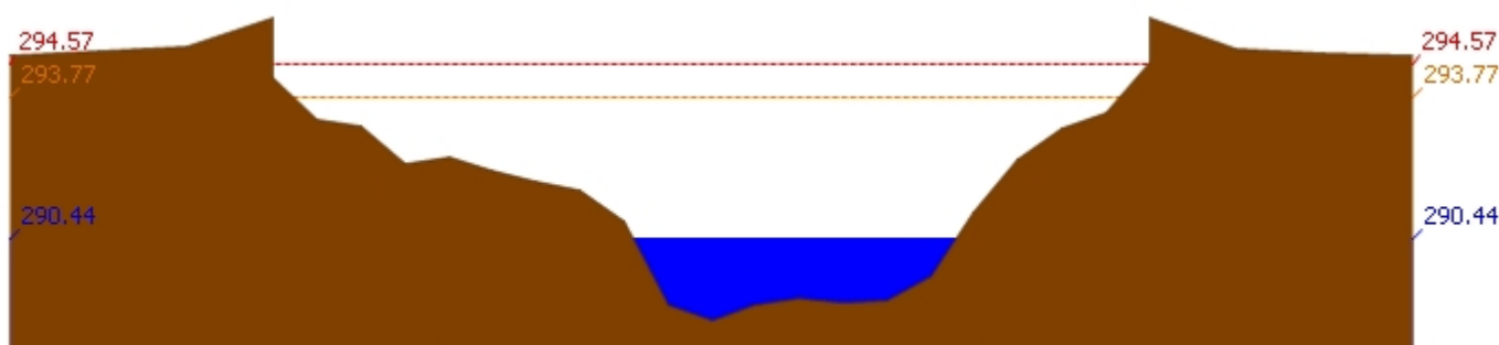
สถานี 060709T น้ำแม่กวงที่ลำพูน ต.เวียงยอง อ.เมือง จ.ลำพูน ระดับน้ำ 290.44 ม.รทก.
