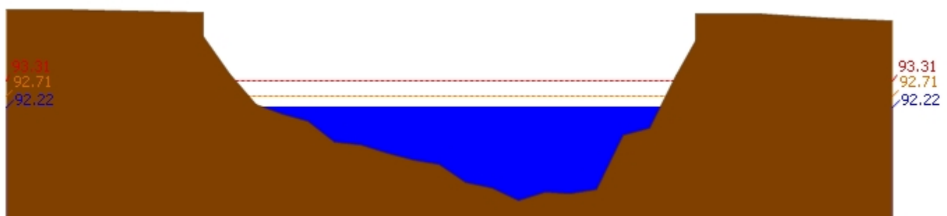
สถานี 061901T คลองแม่ระกาที่บ้านวังชะโอน ต.ท่าไม้ อ.พรานกระต่าย จ.กำแพงเพชร ระดับน้ำ 92.22 ม.รทก.
