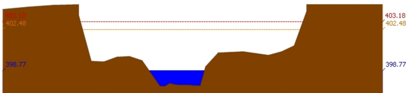
สถานี 060305T น้ำแม่จืดที่บ้านโป่งบัวบาน ต.แม่ป๋อง อ.พร้าว จ.เชียงใหม่ ระดับน้ำ 398.77 ม.รทก.
