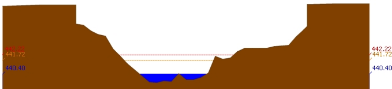
สถานี 060905T น้ำแม่ลี้ที่อำเภอลี้ ต.ลี้ อ.ลี้ จ.ลำพูน ระดับน้ำ 440.40 ม.รทก.
