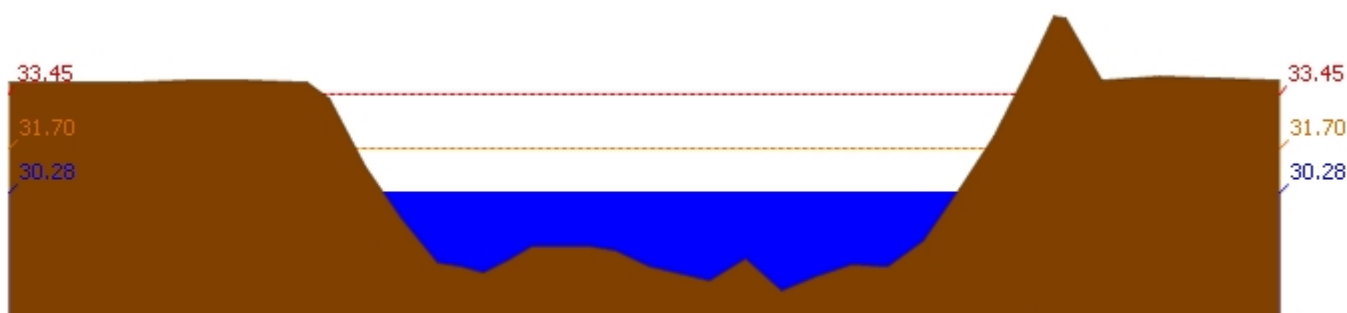
สถานี 110503T แม่น้ำตากแดดที่บ้านหนองขาลาย ต.หนองหลวง อ.สว่างอารมณ์ จ.อุทัยธานี ระดับน้ำ 30.28 ม.รทก.
