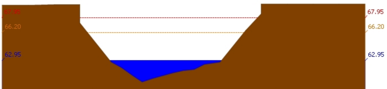
สถานี 110501T น้ำแม่วงก์ที่บ้านคลองสาส์ ต.ลาดยาว อ.ลาดยาว จ.นครสวรรค์ ระดับน้ำ 62.95 ม.รทก.
