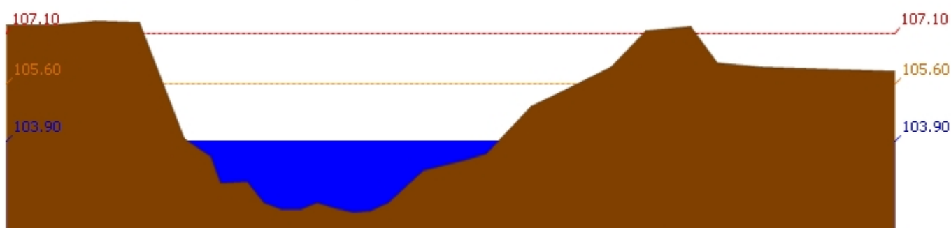
สถานี 110402T ห้วยทับเสลาที่บ้านนาไร่เดียว ต.ลานสัก อ.ลานสัก จ.อุทัยธานี ระดับน้ำ 103.90 ม.รทก.
