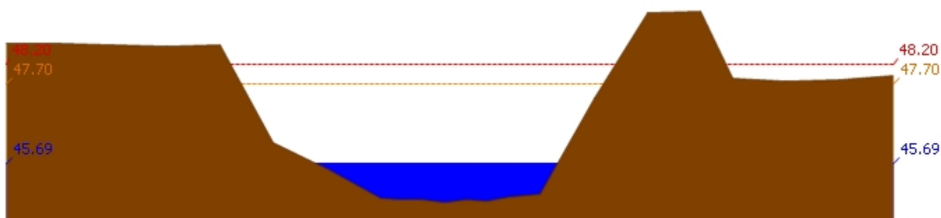
สถานี 110303T คลองโพธิ์ที่บ้านทุ่งสงบ ต.ไม้เขียว อ.สว่างอารมณ์ จ.อุทัยธานี ระดับน้ำ 45.69 ม.รทก.
