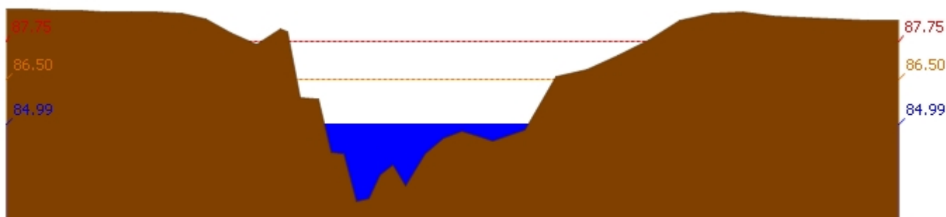
สถานี 110403T ห้วยทับเสลาที่บ้านดินแดง ต.ประดู่ยืน อ.ลานสัก จ.อุทัยธานี ระดับน้ำ 84.99 ม.รทก.
