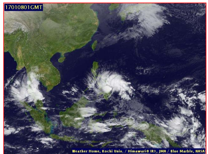
ภาพถ่ายจากดาวเทียม วันที่ ๘ ม.ค. ๒๕๖๐ เวลา ๐๘.๐๐ น.
