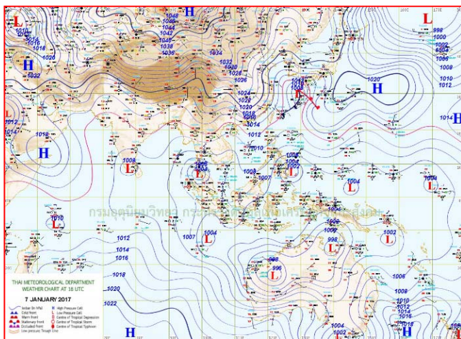
แผนที่อากาศ วันที่ ๘ ม.ค. ๒๕๖๐ เวลา ๐๑.๐๐ น.
