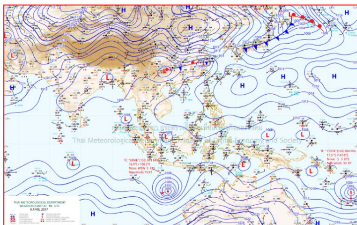
แผนที่อากาศ วันที่ ๙ เม.ย. ๒๕๖๐ เวลา ๐๗.๐๐ น.
