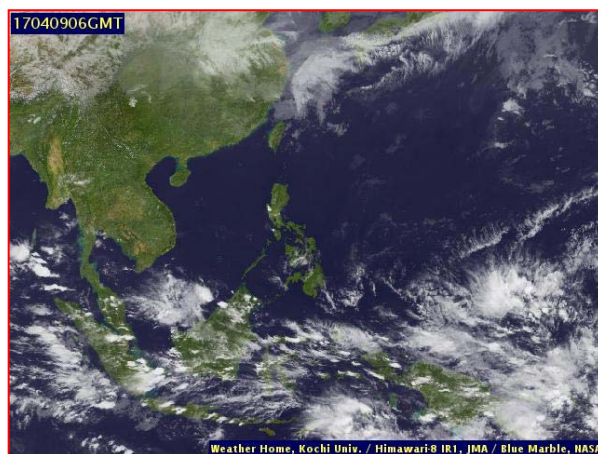
ภาพถ่ายจากดาวเทียม วันที่ ๙ เม.ย. ๒๕๖๐ เวลา ๑๓.๐๐ น.
