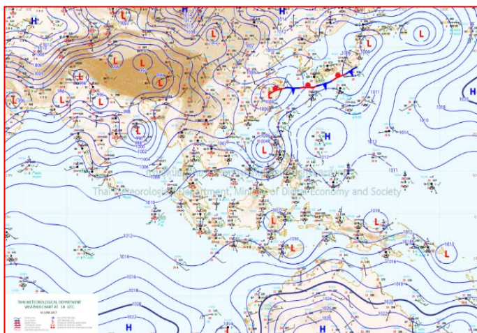
แผนที่อากาศ วันที่ ๑๑ มิ.ย. ๒๕๖๐ เวลา ๐๑.๐๐ น.
