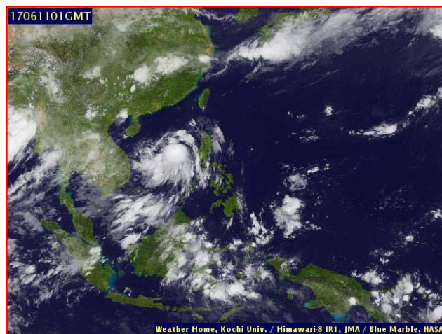
ภาพถ่ายจากดาวเทียม วันที่ ๑๑ มิ.ย. ๒๕๖๐ เวลา ๐๗.๐๐น.
