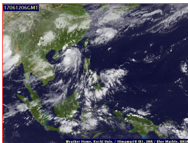
ภาพถ่ายจากดาวเทียม วันที่ ๑๒ มิ.ย. ๒๕๖๐ เวลา ๑๓.๐๐น.
