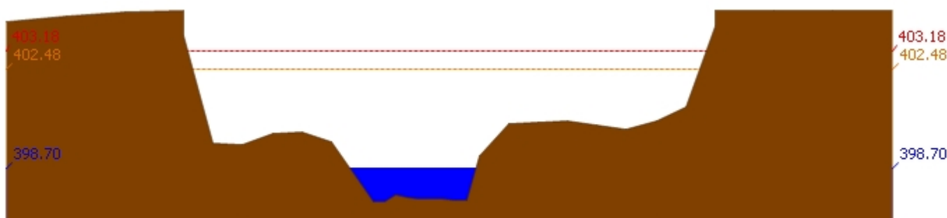
สถานี 060305T น้ำแม่จัดที่บ้านโป่งบัวบาน ต.แม่ป๋อง อ.พร้าว จ.เชียงใหม่ ระดับน้ำ 398.70 ม.รทก.
