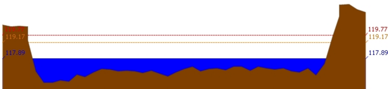
สถานี 060111T แม่น้ำปิงที่บ้านปากร่องห้วยจี้ ต.ตากออก อ.บ้านตาก จ.ตาก ระดับน้ำ 117.89 ม.รทก.
