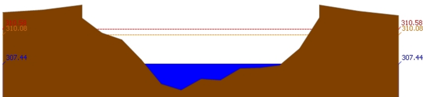
สถานี 060814T น้ำแม่ขานที่บ้านท่าโป่ง ต.บ้านแม่ อ.สันป่าตอง จ.เชียงใหม่ ระดับน้ำ 307.44 ม.รทก.
