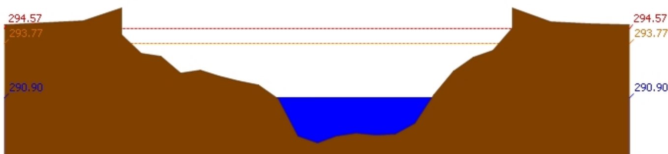
สถานี 060709T น้ำแม่กวงที่ลำพูน ต.เวียงยอง อ.เมือง จ.ลำพูน ระดับน้ำ 290.90 ม.รทก.
