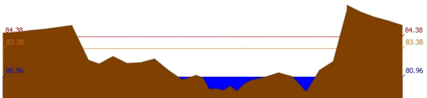
สถานี 062001T คลองสวนหมากที่บ้านน้ำไทรง ต.ท่าขุนราม อ.เมือง จ.กำแพงเพชร ระดับน้ำ 80.96 ม.รทก.
