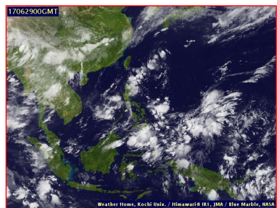
ภาพถ่ายจากดาวเทียม วันที่ 29 มิ.ย. 2560 เวลา 07.00 น.
