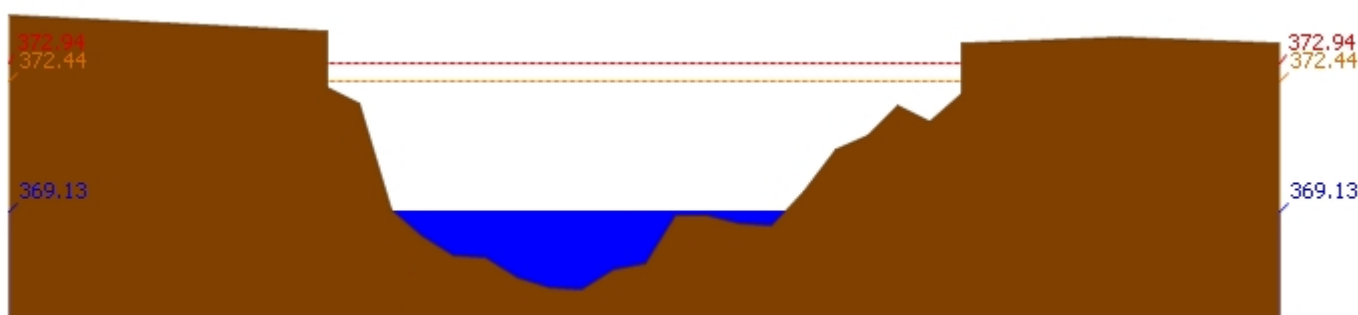
สถานี 060109T แม่น้ำปิงที่บ้านสบฮ้อย ต.แม่ระ อ.เชียงดาว จ.เชียงใหม่ ระดับน้ำ 369.13 ม.รทก.
