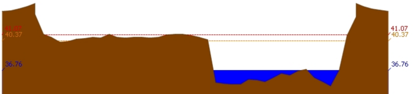
สถานี 060110T แม่น้ำปิงที่บ้านบางแก้ว ต.บางแก้ว อ.บรรพตพิสัย จ.นครสวรรค์ ระดับน้ำ 36.76 ม.รทก.
