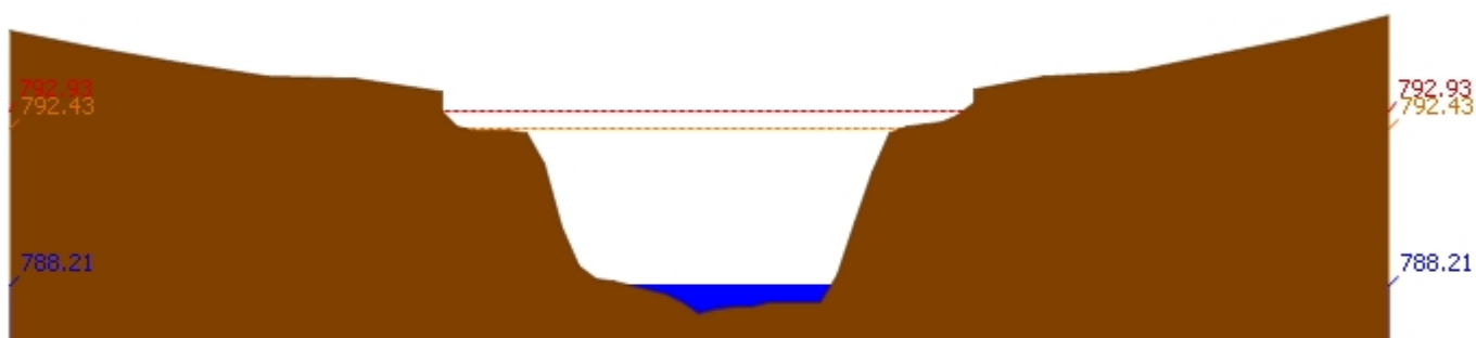
สถานี 061503T น้ำแม่ต้นที่บ้านคอย ต.ยางเปียง อ.อมก๋อย จ.เชียงใหม่ ระดับน้ำ 788.21 ม.รทก.
