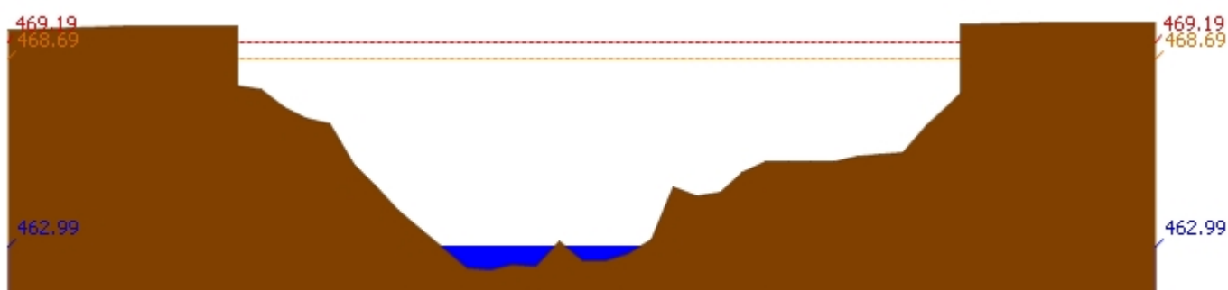
สถานี 060905T น้ำแม่ลี้ที่อำเภอลี้ ต.ลี้ อ.ลี้ จ.ลำพูน ระดับน้ำ 462.99 ม.รทก.
