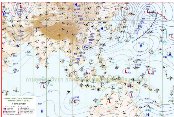
แผนที่อากาศ วันที่ ๓๑ ม.ค. ๒๕๖๐ เวลา ๐๗.๐๐ น.
