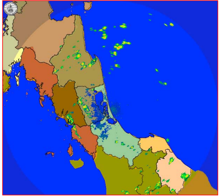
สถานีสงขลา เวลา ๑๔.๓๐ น.
